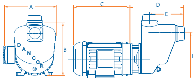
MODELOS: 722 / 725
